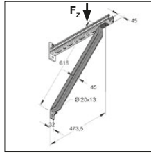
Zastrzał 45° długi
