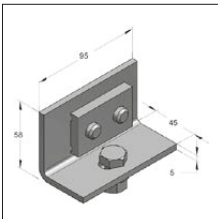
Wspornik adaptera
