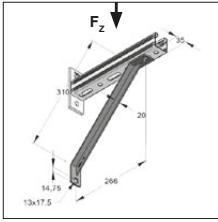
Zastrzał 45° krótki
